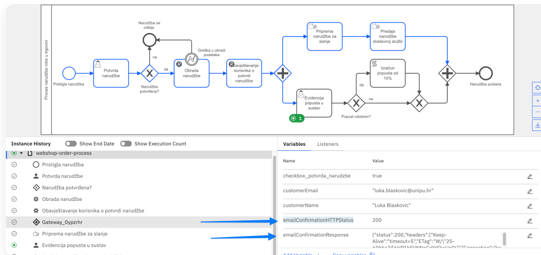
Slika 22. U Camunda Operate aplikaciji možemo vidjeti da je otpremni zadatak "Obavješćavanje korisnika o potvrdi narudžbe" uspješno izvršen.
