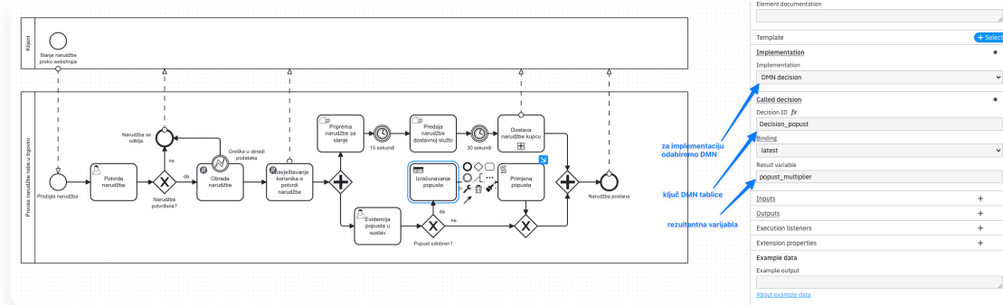
Slika 30. Dodavanje Business Rule Task a za povezivanje s DMN tablicom odluka.
