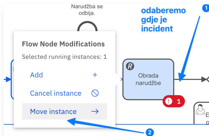
Slika 10. Unutar Camunda Operate aplikacije odaberite Modify Instance, a potom Move instance da biste preusmjerili tok procesa na drugu aktivnost.
