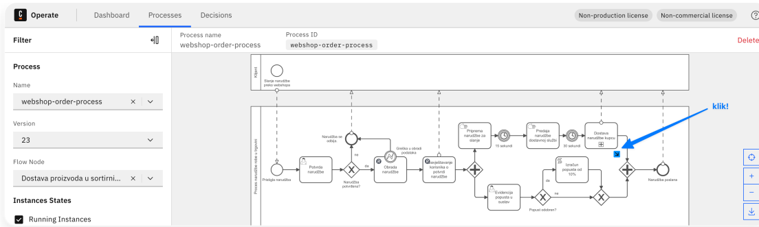
Slika 27. Pregled potprocesa unutar Camunda Operate aplikacije.
