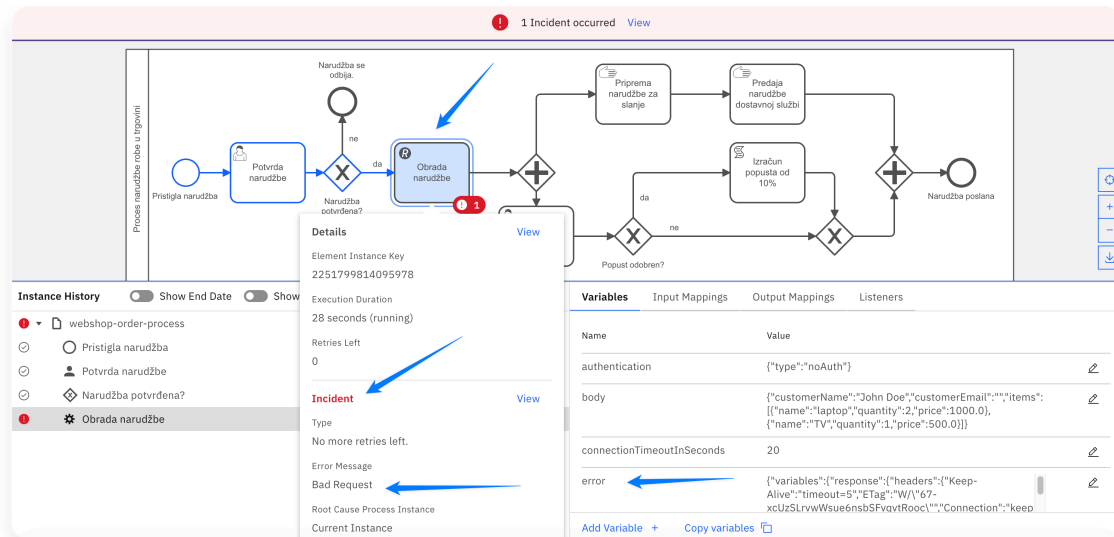
Slika 8. U slučaju greške (npr. nedostaje email adresa kupca), servisni zadatak "Obrada narudžbe" će pasti s greškom jer nismo implementirali rukovanje greškama.
