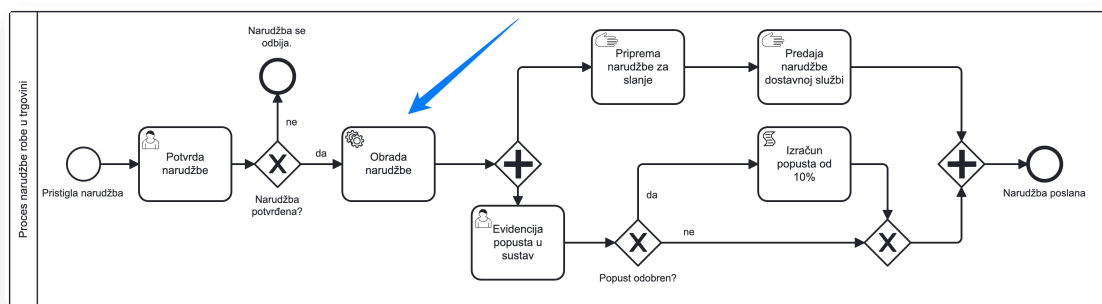
Slika 2. Servisni zadatak "Obrada narudžbe" dodajemo nakon "da" slijeda iz skretnica "Narudžba potvrđena?".
