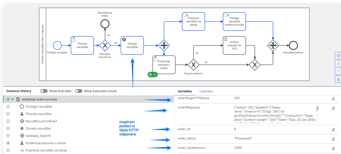
Slika 7. Unutar Camunda Operate aplikacije možemo vidjeti mapirane podatke iz HTTP odgovora pohranjene u procesne varijable nakon izvršenja servisnog zadatka "Obrada narudžbe".
