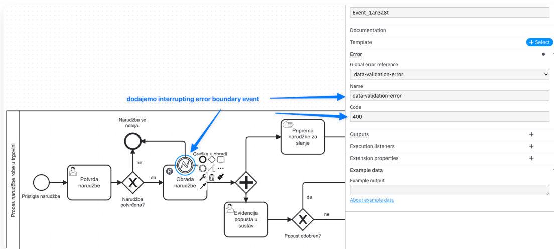
Slika 12. Konfiguracija interrupting error boundary eventa za hvatanje greške s kodom 400.
