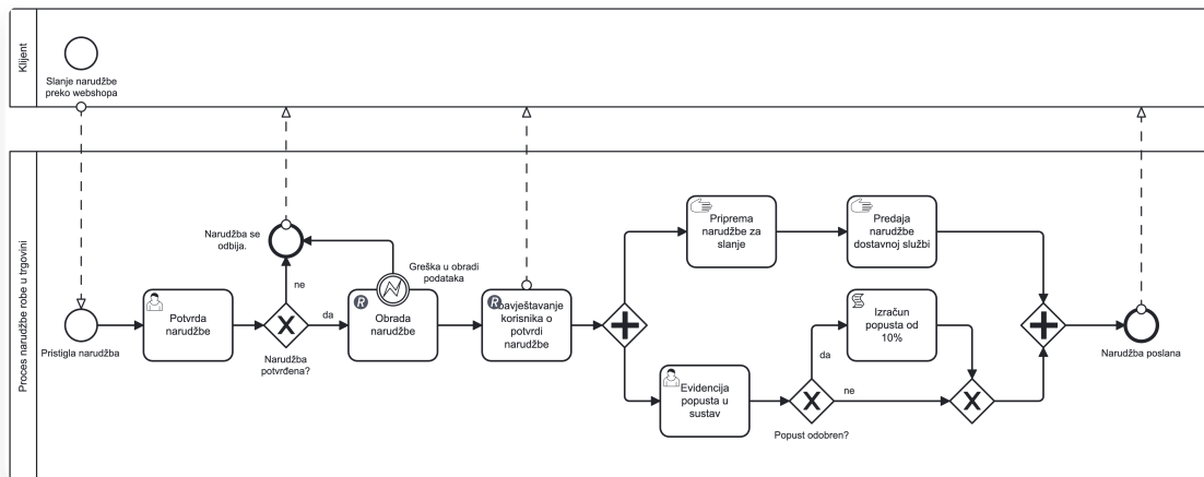
Slika 23. Dodavanje apstraktnog polja "Klijent" i informacijskih tokova između procesne aplikacije i klijenta.
