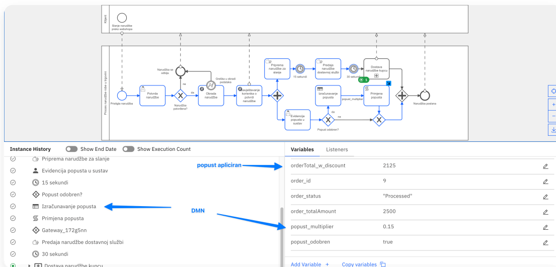
Slika 32. Primjer izvršavanja procesa u Operateu gdje je DMN tablica odlučila o visini popusta na temelju ukupnog iznosa narudžbe.
