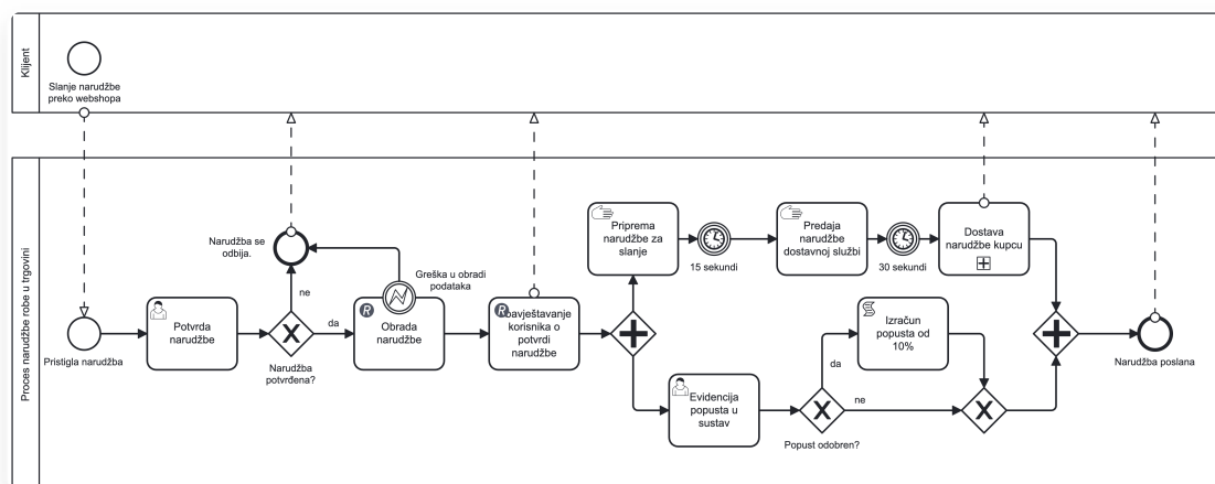
Slika 26. Cjelokupni BPMN dijagram procesne aplikacije za upravljanje narudžbama s dodanim potprocesom "Dostava narudžbe kupcu".
