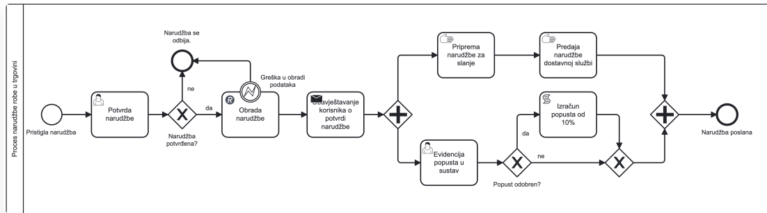
Slika 14. Dodavanje otpremnog zadatka "Obavješćivanje korisnika o potvrdi narudžbe" nakon servisnog zadatka "Obrada narudžbe".
