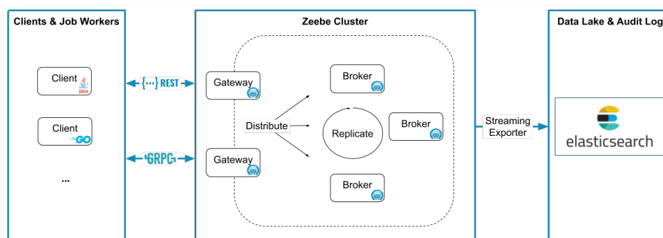
Slika 1. Arhitektura Camunda 8 Zeebe procesnog enginea (izvor: Camunda Documentation )
