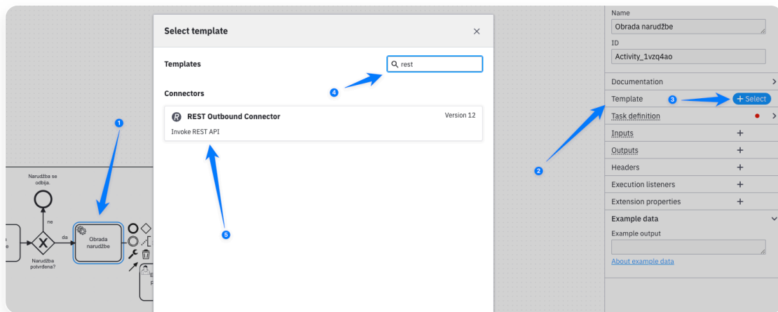
Slika 6. Odabir REST Outbound Connectora u postavkama servisnog zadatka.
