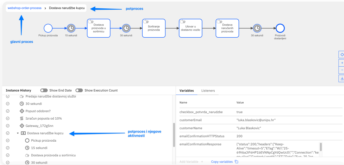
Slika 28. Praćenje izvršavanja instance potprocesa unutar Camunda Operate aplikacije.
