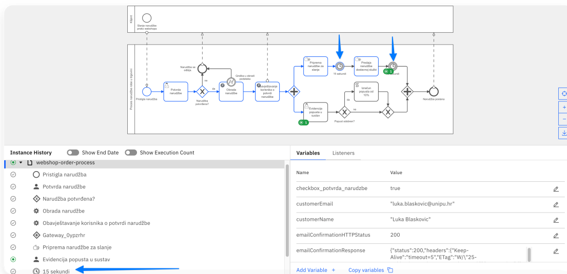
Slika 24. Dodavanje intermediate timer eventa za simulaciju trajanja aktivnosti nakon ručnih zadataka.
